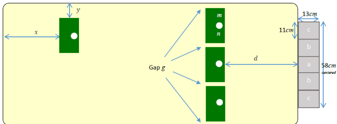
图 2——场地尺寸图
